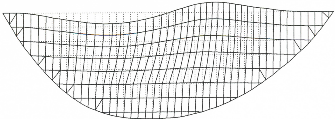
図-3 表層地盤の1次卓越振動モード
