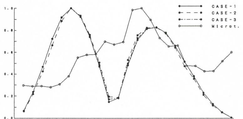
図-4 上下動応答値の分布に関する比較
