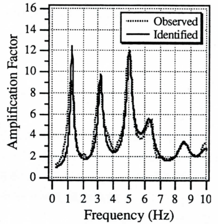
図-2 同定モデルの伝達関数
