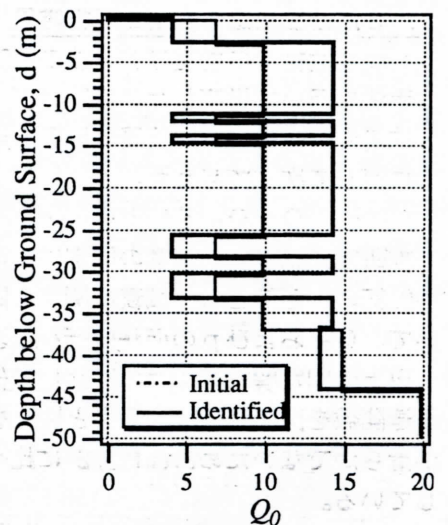
図-4 Q_0 値の同定結果
