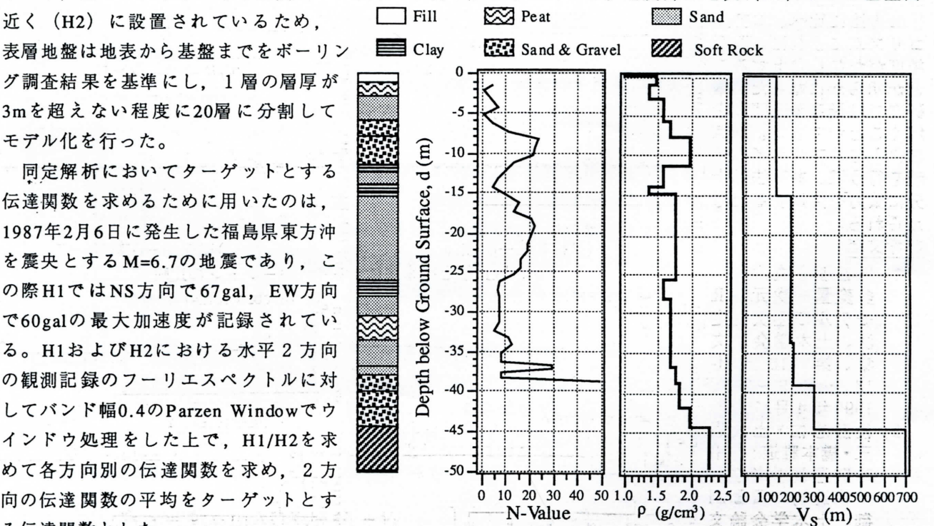
図-1 KASSEMセンターアレーH12地点の土質プロファイル
