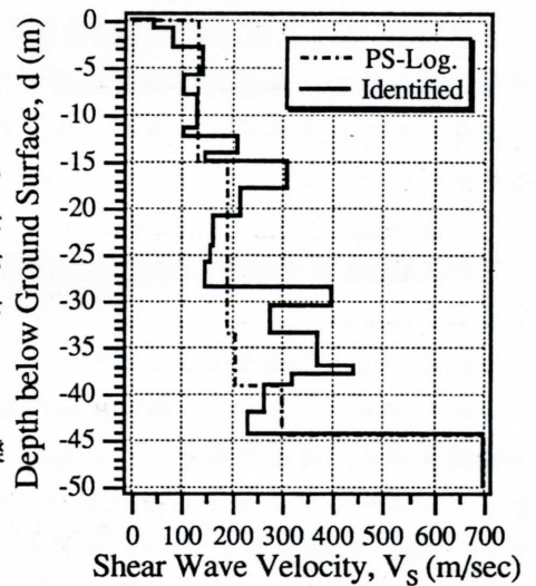
図-3 せん断波速度の同定結果
