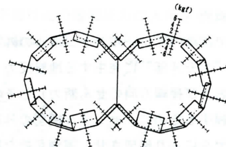
図9 法線方向最大地盤反力分布（複円）
