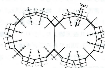
図7 接線方向最大せん断力分布（複円）
