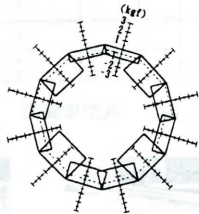
図8 法線方向最大地盤反力分布（単円）
