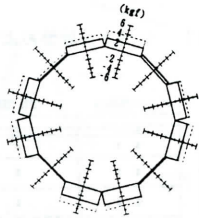
図6 接線方向最大せん断力分布（単円）
